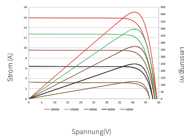
Strom-Spannungs- und Leistungs-Spannungs-Diagramme(615W)
